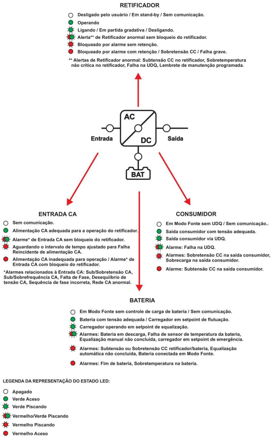
Figura 7 - SINÓTICO OPERACIONAL - REPRESENTAÇÃO LEDS
