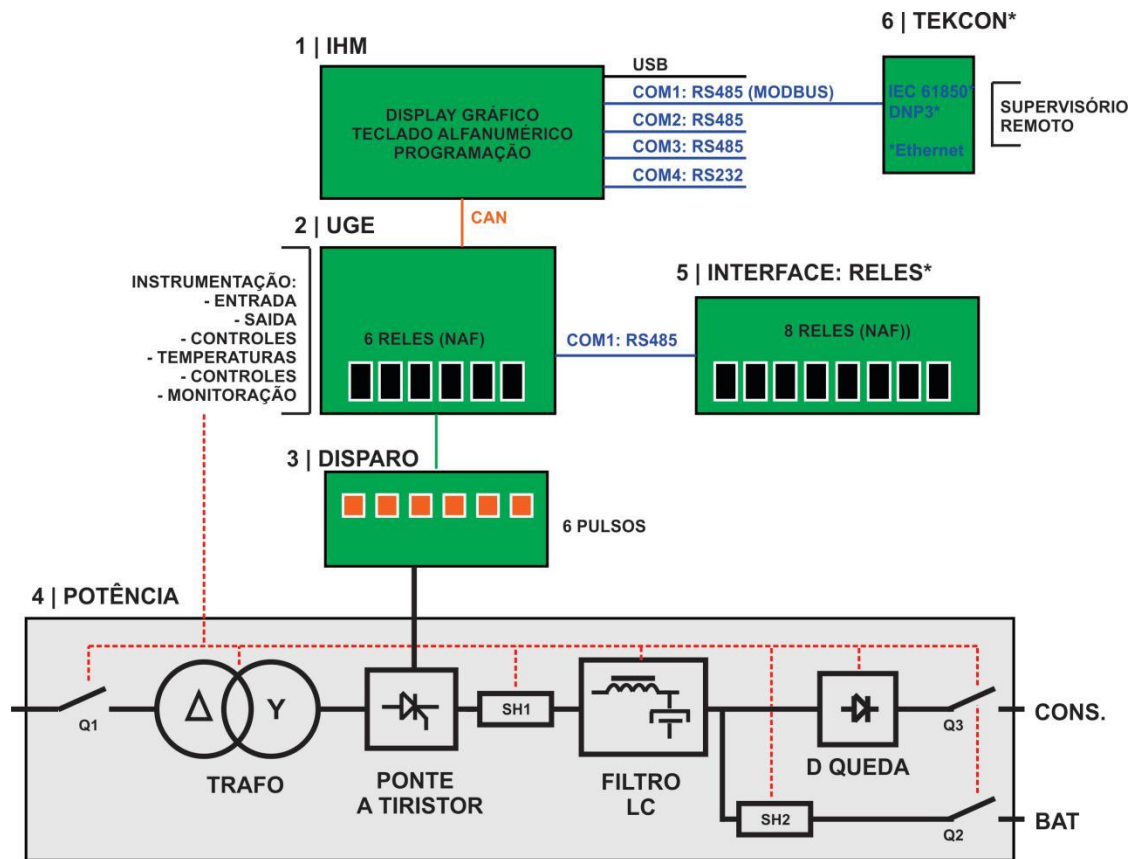
Figura 3 - Versão de 6 Pulsos
