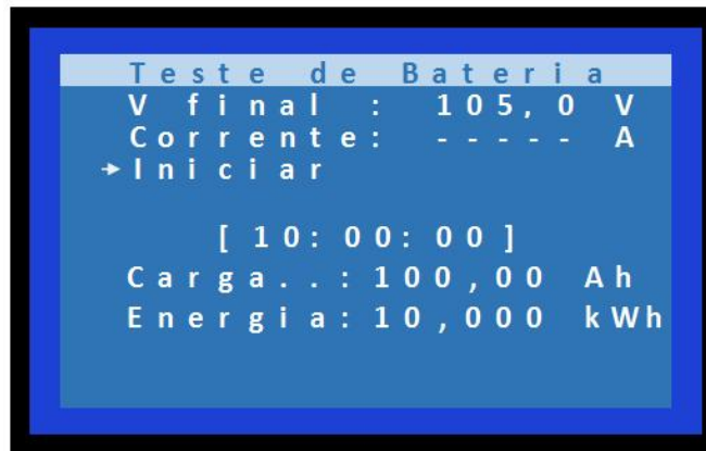
Figura 16 - Medições do Teste de Baterias
