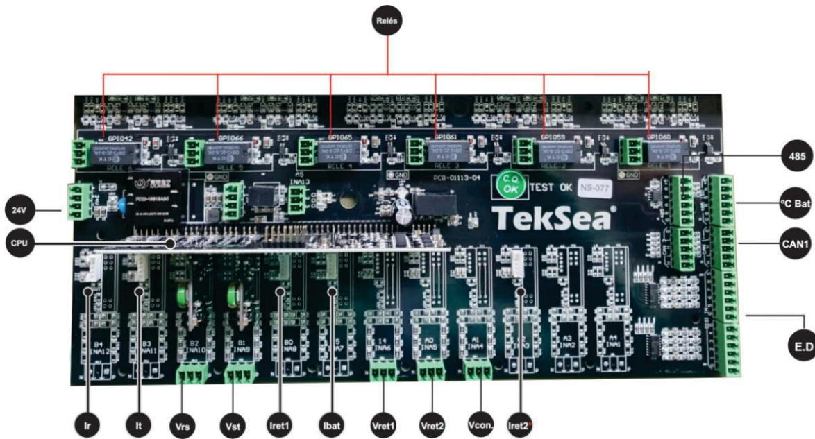
Figura 9 - Unidade de Gerenciamento de Energia - UGE
