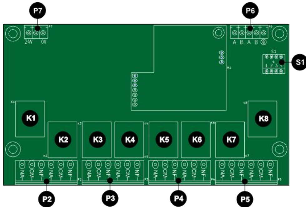
Figura 11 - Interface de Expansão - Cartão de Relés
