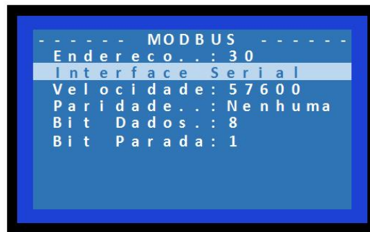
Figura 17 - Parâmetros Modbus RTU
