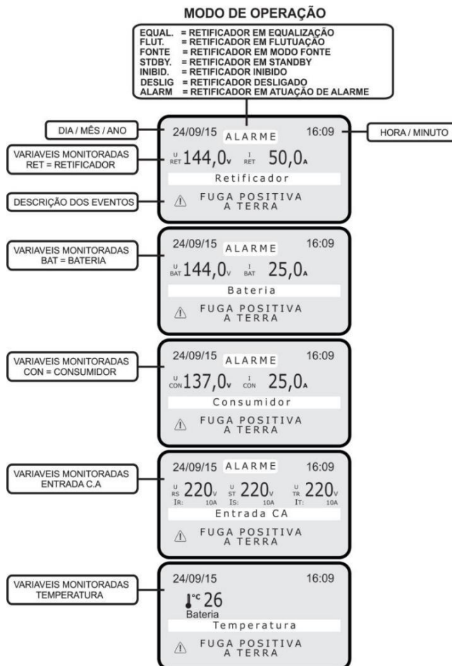
Figura 8 - Display Gráfico
