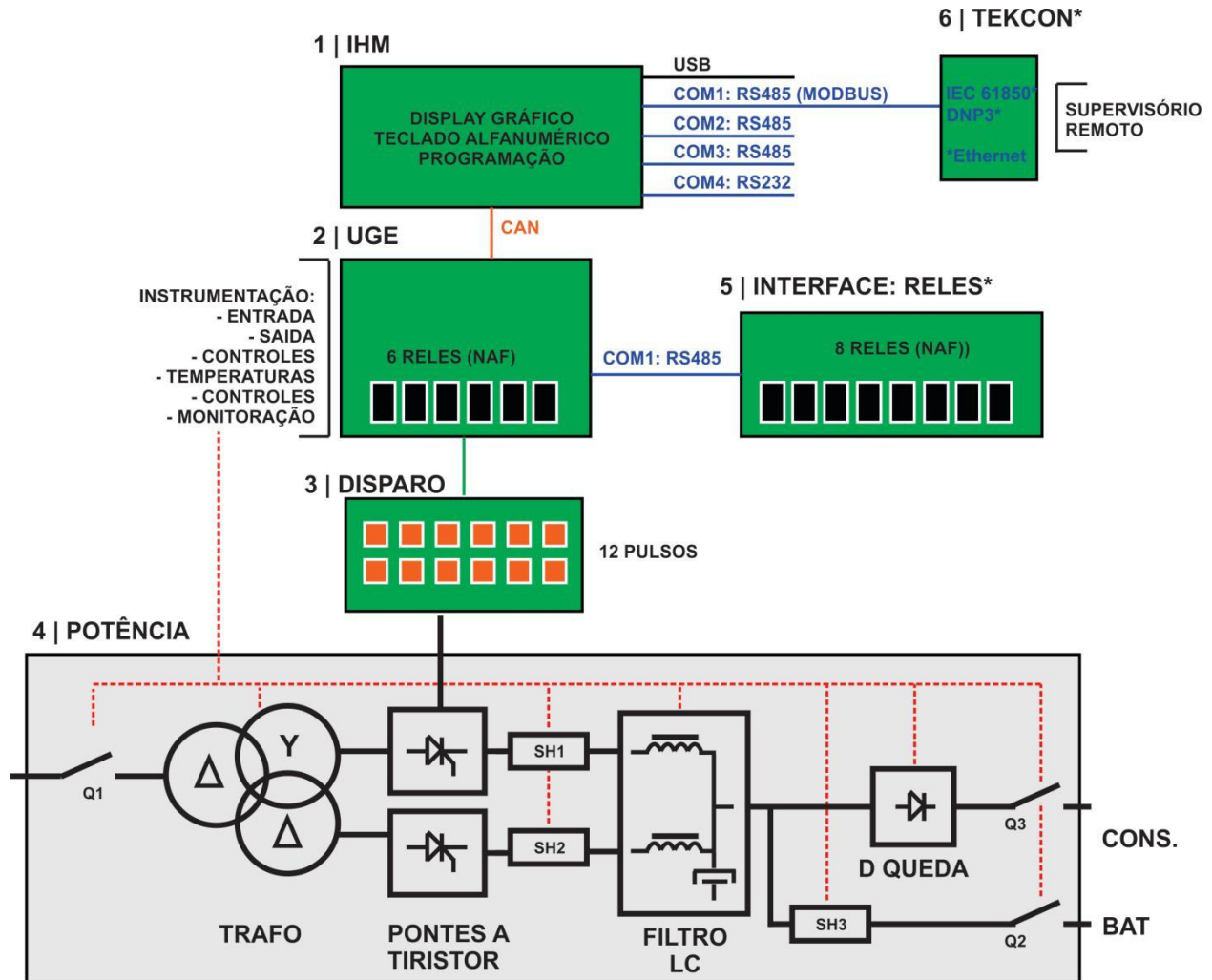
Figura 4 - Versão de 12 Pulsos
