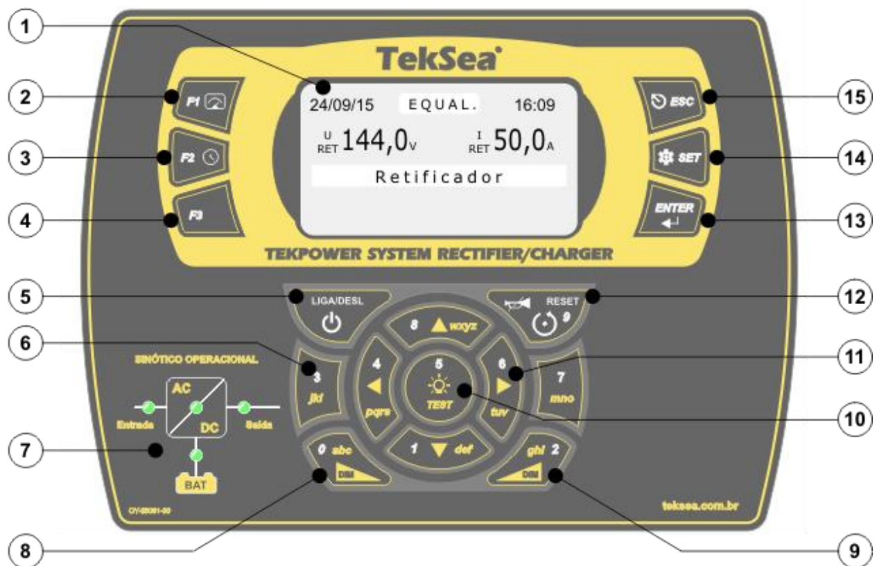
Figura 5 - IHM 6/12 PULSOS
