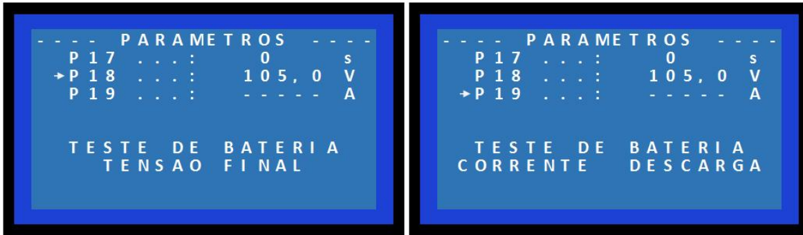
Figura 13 - Parâmetros - Teste de Baterias
